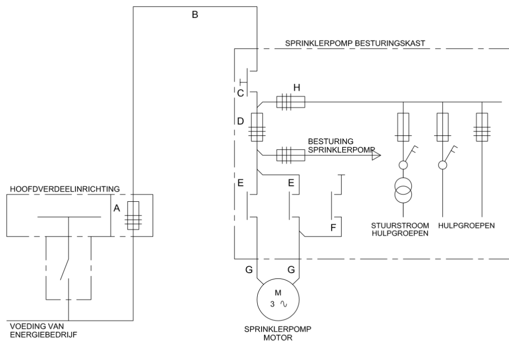
● Figuur 10.1.5.4-1: Schema sprinklerpomp met onderbeveiliging.
