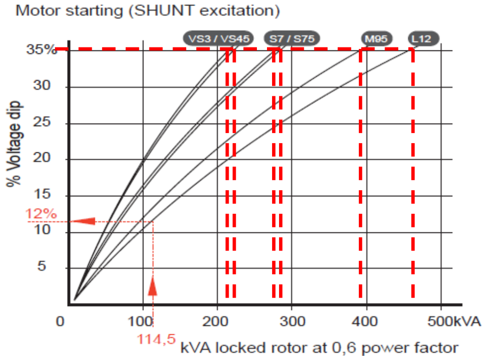
Afbeelding .6 Shunt bekrachtiging
