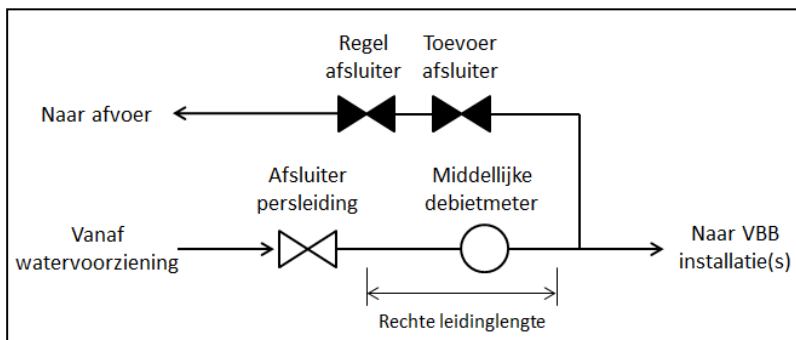
Figuur 4.4.1.1-2: waterloopschema debietmeter in de toevoerleiding
