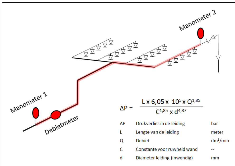
Figuur T4.4.1.3: bepalen C-waarde tussen manometers
