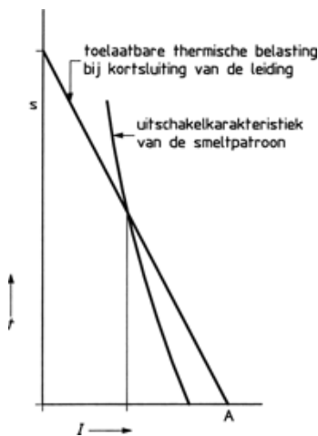
Figuur 10.2.8-1: Het verband tussen de uitschakelkarakteristiek van de smeltpatroon en de toelaatbare thermische belasting bij kortsluiting van de leiding.
