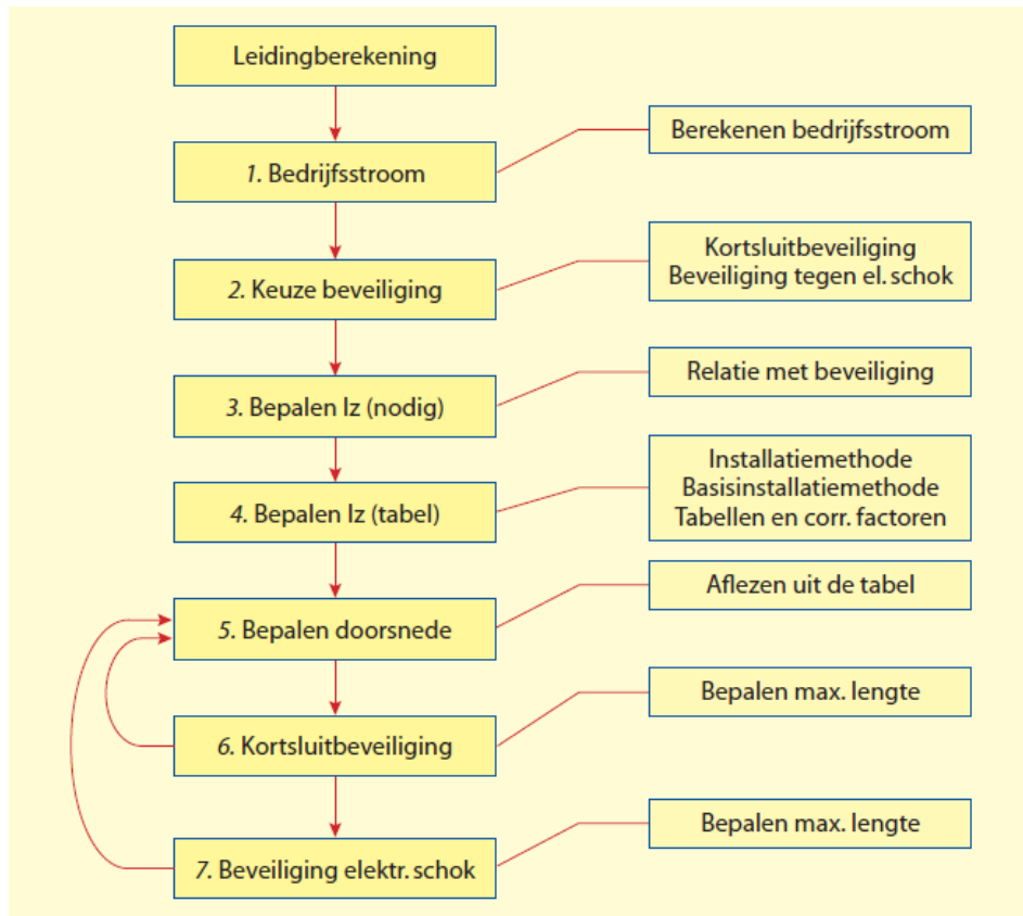
Figuur 10.2.9: Stappenplan voor het berekenen van leidingdoorsneden.
