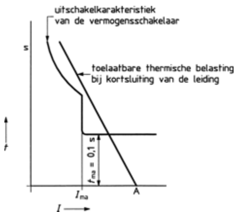
Figuur 10.2.8-2: Het verband tussen de uitschakelkarakteristieken van de vermogensschakelaar en de toelaatbare thermische belasting bij kortsluiting van de leiding.
