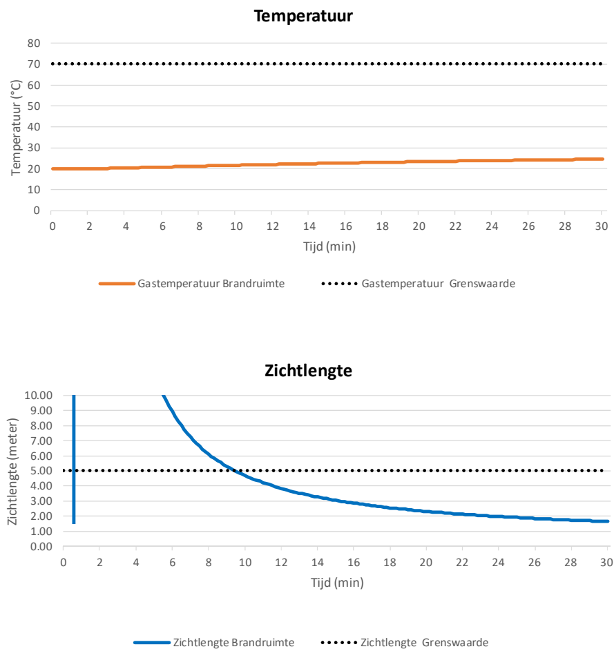
Figuur 11: Simulatieresultaat grote lage ruimte, gesprinklerde situatie, toetsing criterium gezondheidsschade
