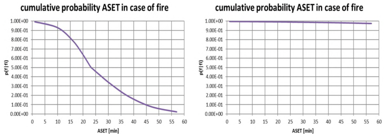
Figuur 9: Cumulatieve kansverdeling ASET in de grote hoge ruimte, criterium gezondheidsschade – rookvrije hoogte > 2,5 m (links: ongesprinklerde referentiesituatie; rechts: gespreinklerde situatie)
